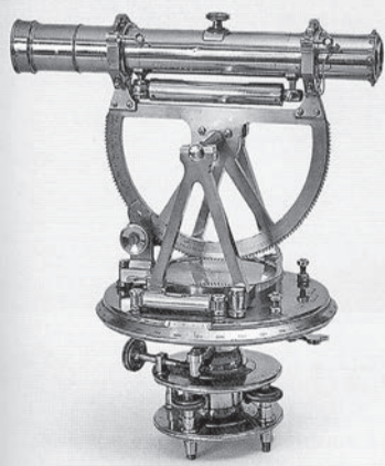
Теодолит 1840 г.
